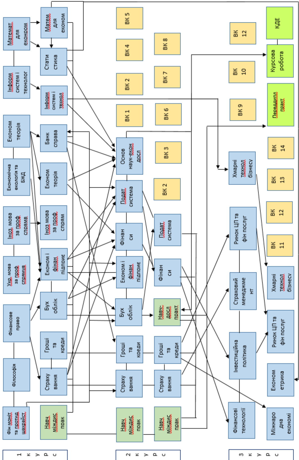
Структурно-логічна схема
